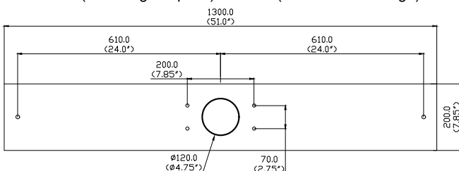
Cardboard (mounting template) / Carton (modèle de montage)
