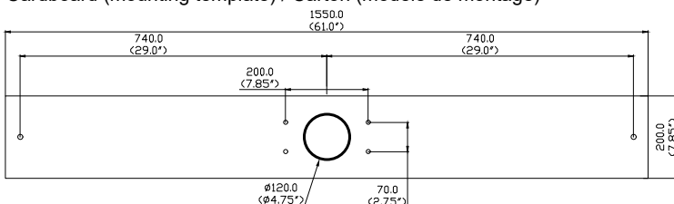
Cardboard (mounting template) / Carton (modèle de montage)
