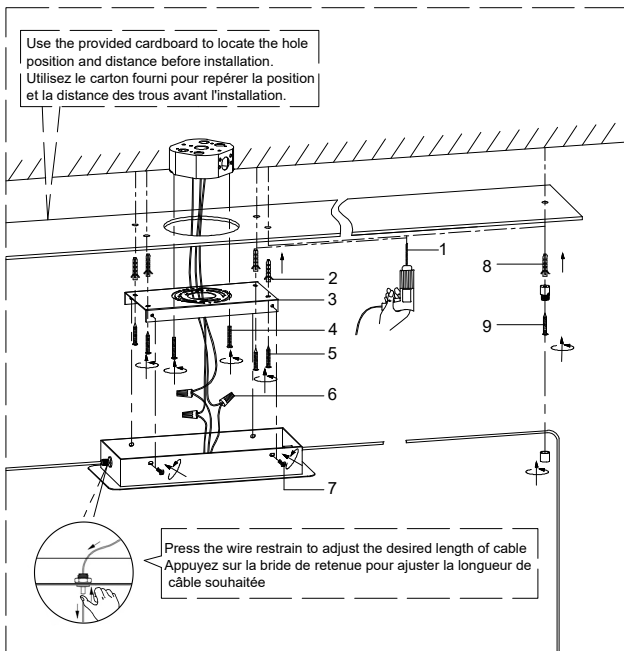
Assembling glass / Assemblage du verre
